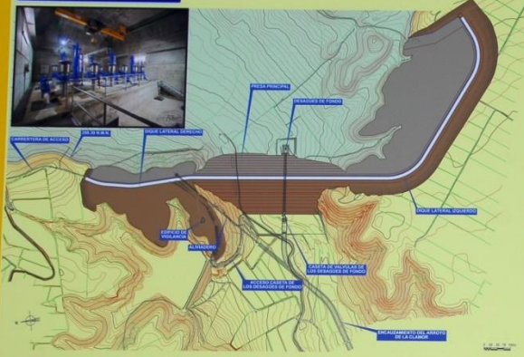
PLANTA GENERAL DE LA PRESA
