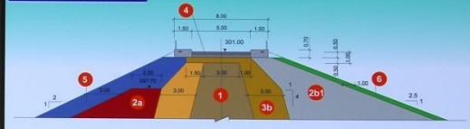
DETALLE DE CORONACIÓN
