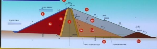
SECCIÓN TIPO EN CAUCE (P1/P5 Y P9/P14)
